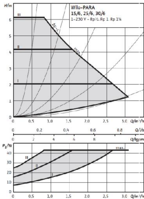
Diferencial de presión constante ( P=c )
