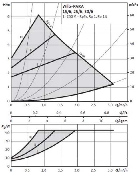
Diferencial de presión variable ( P=v )
