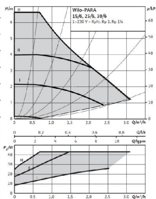
Velocidad constante ( P=c )
